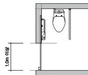
그림 23. 화장실 출입문 유효폭 규정
