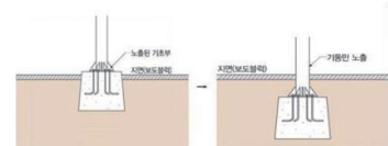
그림 75. 지지대와 앵커볼트의 매립을 통한 미려한 지면 결합 부위 마감 처리
